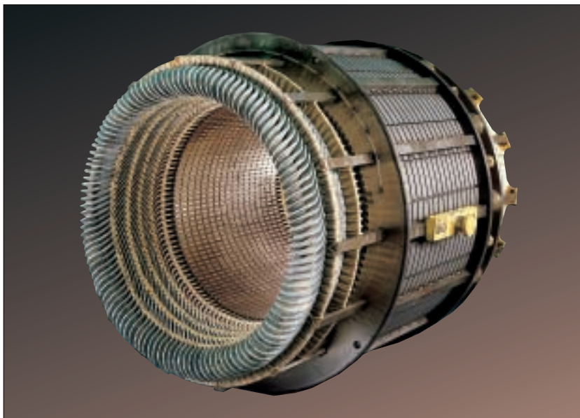
Ständerblechpaket mit Wicklung
