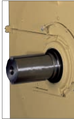
Wälzlager mit Nachschmiereinrichtung und Fettentnahmevorrichtung
